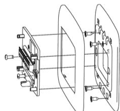
Deux coffrets (carré de 4 po) électriques (plaque murale vendue séparément)
