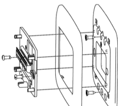
Coffret électrique seul vertical (plaque murale vendue séparément)
